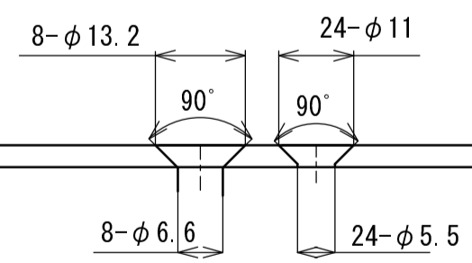
断面A-A
