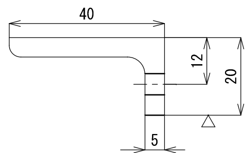
断面A-A
