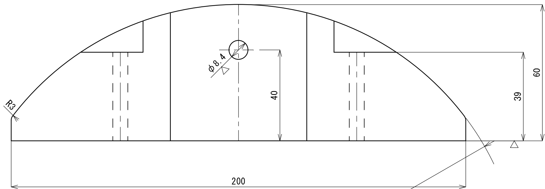
断面A-A
