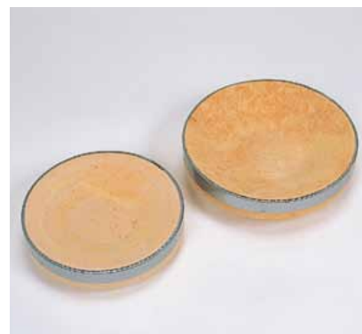
54KI 0006 燃焼台 大 (φ260×H80)1入 燃焼台 小 (φ240×H60)1入
